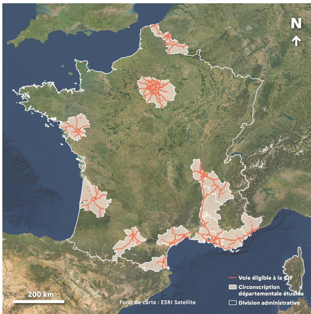
Illustration 4 – Les réseaux routiers adéquats à la circulation inter-files
